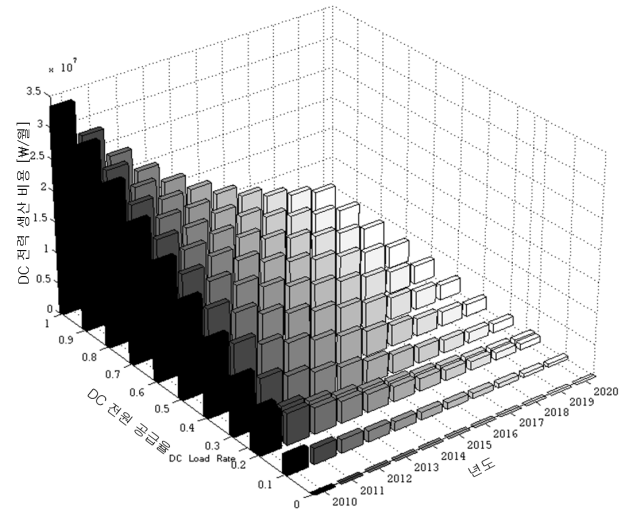
그림 6 DC 전원 공급율에 따른 연간 DC 전력 공급 비용 Fig. 6 Annual DC power supply cost according to the ratio of DC power supply
