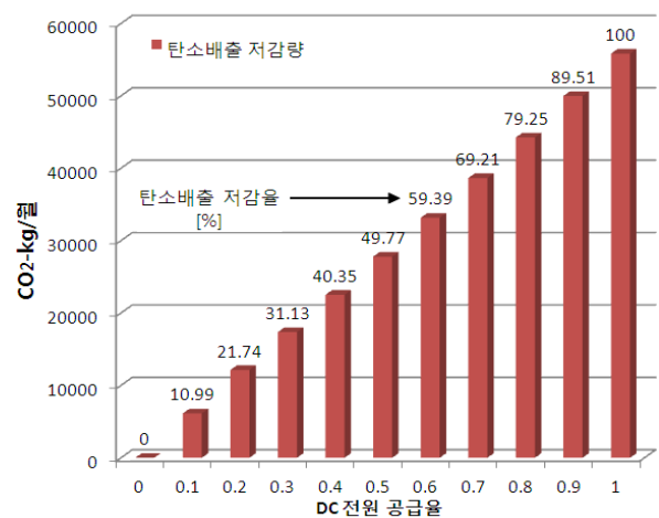
그림 4 DC 전원 공급율에 따른 탄소배출 저감량
