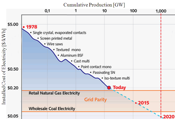
그림 3 태양광 발전의 Grid Parity Fig. 3 Grid Parity for solar energy
