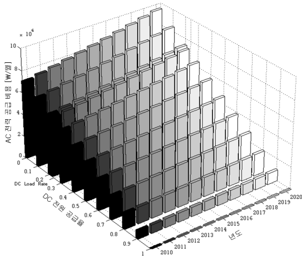
그림 5 DC 전원 공급율에 따른 연간 AC 전력 공급 비용 Fig. 5 Annual AC power supply cost according to the ratio of DC power supply
