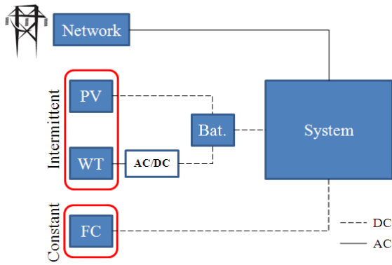
그림 2 신재생에너지를 통한 DC 전원 공급 개념도 Fig. 2 Energy supply concept with DC power system having renewable energies
