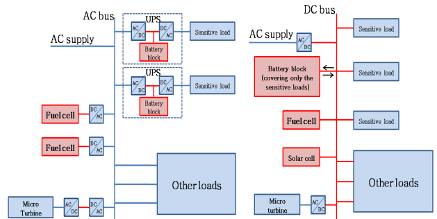
그림 1 AC 배전 방식 vs DC 배전 방식 Fig. 1 AC Distribution vs DC Distribution
