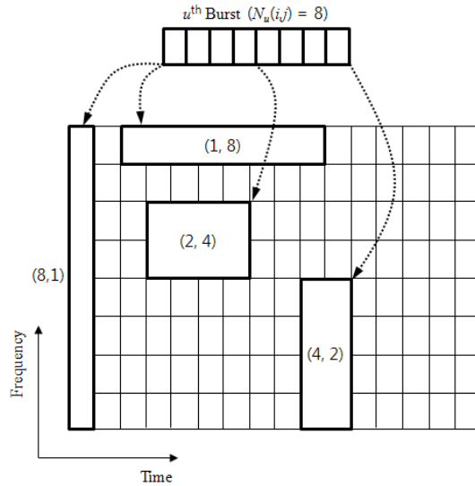
그림 4. 시간-주파수 축에서의 Burst 할당 예 Fig. 4. Example of burst allocation in time-frequency axis
