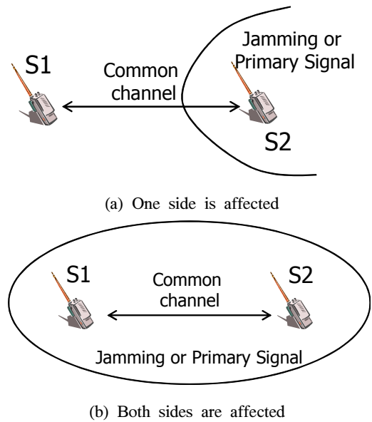
그림 5. 두 무전기가 통신하고 있는 채널에 주 사용자가 나타나거나 재밍 공격이 발생한 경우 Fig. 5. Occurrence of jamming attack or PU signal on common channel
