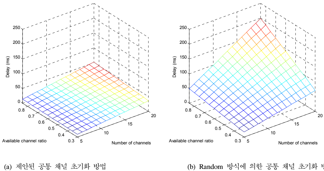
그림 12. N_C 와 R_{AC} 의 변화에 따른 공통 채널 초기화 과정의 지연 시간 ( SM=0.75 , R_{PL}=0.055 ) Fig. 12. Common channel initialization setup delay according to different N_C and R_{AC}
