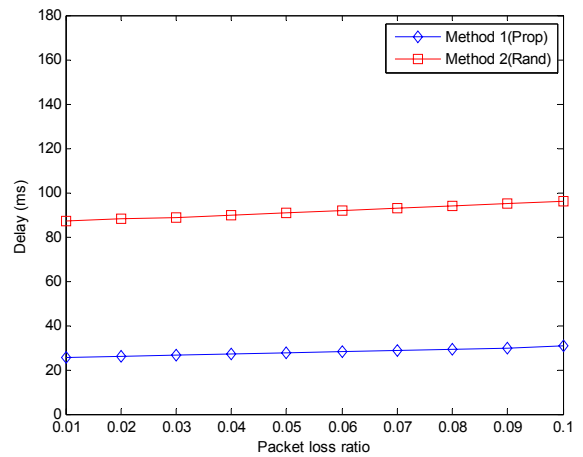
(d) T_{CCRD} vs. R_{PL} ( N_C=12 , R_{AC}=0.65 , SM=0.75 )
