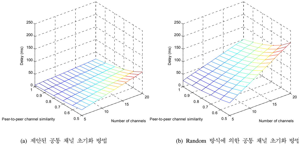
그림 11. N_C 와 SM 의 변화에 따른 공통 채널 초기화 과정의 지연 시간 ( R_{AC}=0.65 , R_{PL}=0.055 ) Fig. 11. Common channel initialization setup delay according to different N_C and SM
