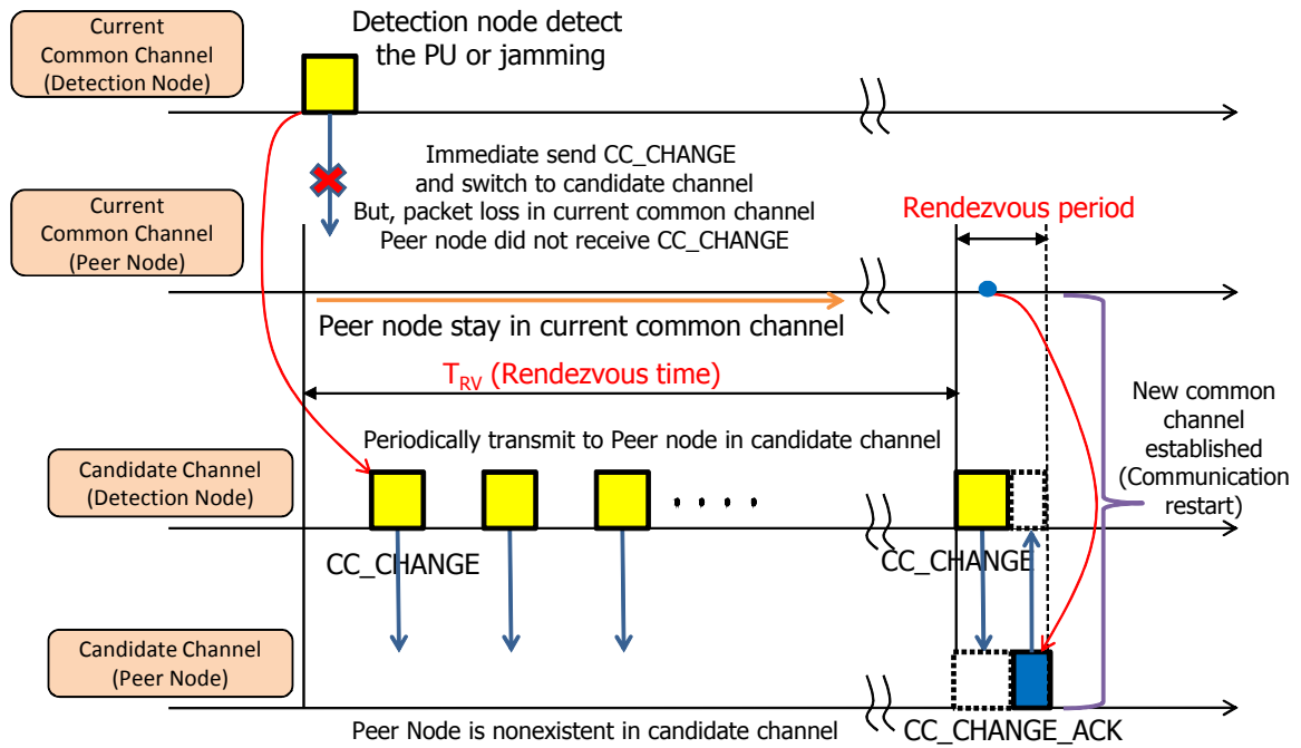
그림 7. 란데부 시간에 의한 공통 채널 복원 과정 Fig. 7. Common channel reconstruction procedure by rendezvous time
