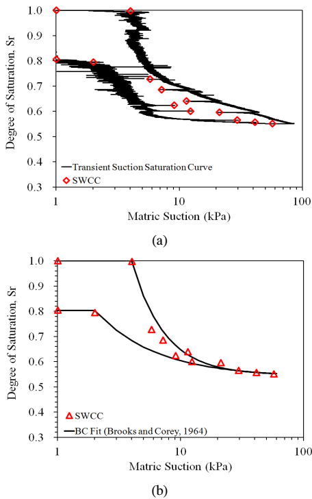
[그림 10] 비정상 흡입력-포화도 곡선 및 함수특성곡선 (화강풍화토) [Fig. 10] Transient suction-saturation curve and SWCC(Weathered granite)
