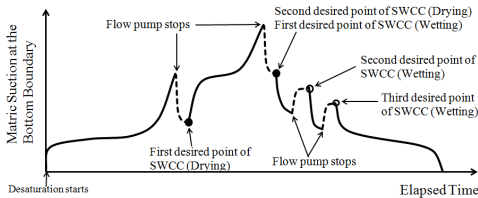
[그림 5] 흡입력 조절 기법의 원리 [Fig. 5] Principle of suction control technique
