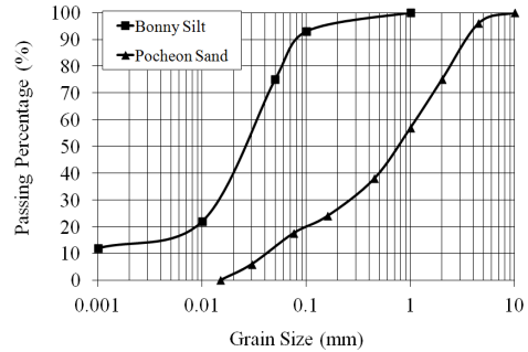
[그림 6] 실험시료의 입도분포곡선 [Fig. 6] Grains size distribution of two sands
