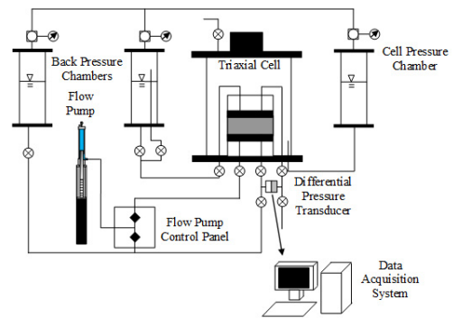
[그림 1] 플로우 펌프 시스템 모식도[7]
