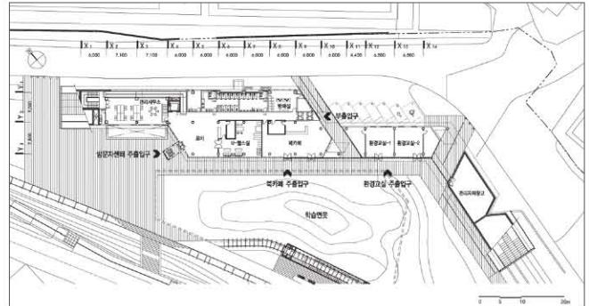
1층 평면도
