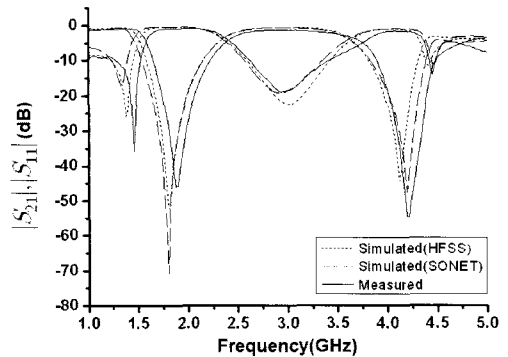
그림 6. 대역 저지 필터의 특성 Fig. 6. Characteristics of Band Stop Filter
