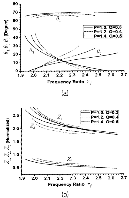
그림 4. r_f 에 대한 선로의 길이와 임피던스 (a) r_f 에 대한 \theta_1, \theta_2 및 \theta_3 (b) r_f 에 대한 임피던스 Z_1, Z_2, Z_3 Fig. 4. Line Length and Impedance for r_f (a) \theta_1, \theta_2, \theta_3 for r_f (b) Z_1, Z_2, Z_3 Impedance for r_f
