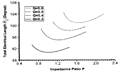
그림 3. TSSIR의 P와 Q에 대한 선로의 길이 \theta_L Fig. 3. Line Length \theta_L for P and Q of TSSIR
