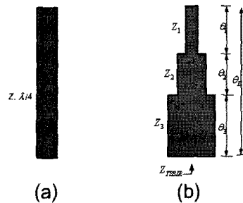
그림 1. 마이크로 스트립 선로 공진기 (a) \lambda/4 스텐브 (b) 3단 계단형 임피던스 공진기 Fig.1 Microstrip Line resonator (a) \lambda/4 Stub (b) Tri-step Impedance Resonator
