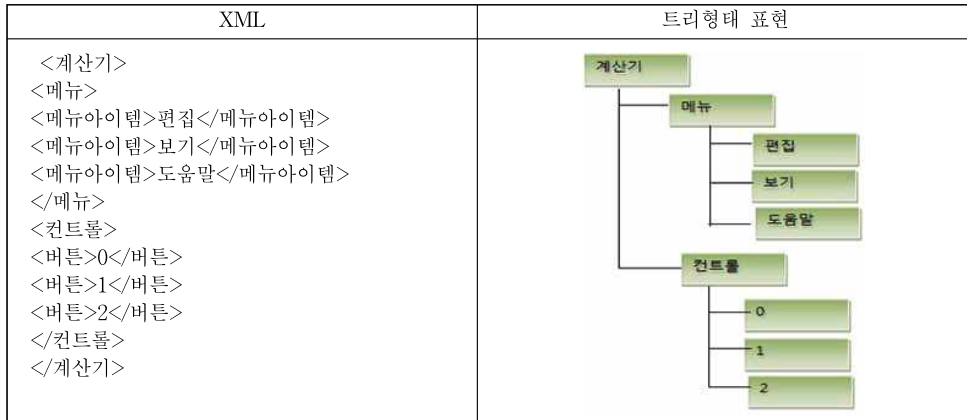
(그림 2) GUI MAP의 예
