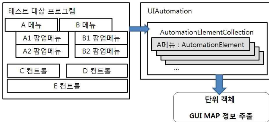
(그림 1) UIAutomation을 이용한 단위 객체 정보 추출
