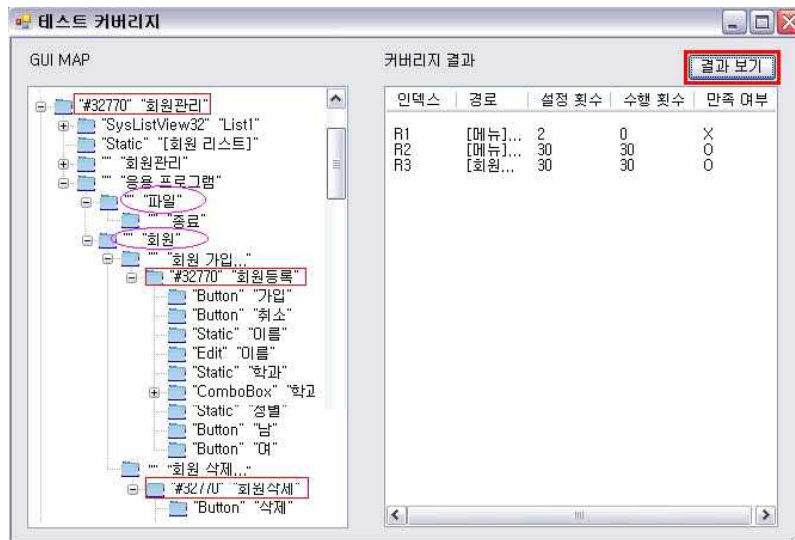
(그림 8) 테스트 커버리지 결과
