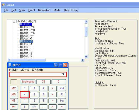
(그림 3) UI Automation을 이용한 단위 객체 추출
