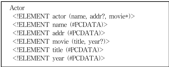
(그림 1) Actor DTD
