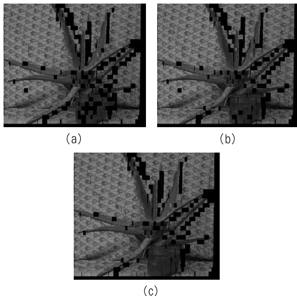
(그림 7) 좌 영상으로부터 우 영상을 블록단위로 움직임을 추정하고 매핑을 한 결과: (a) 영상 정규화 (b) 히스토그램 명세화 (c) 제안된 방법
