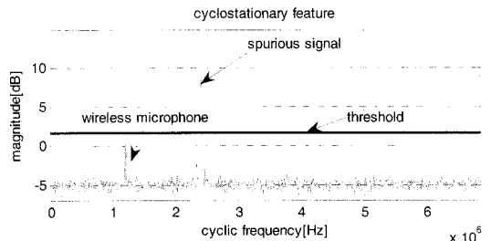
그림 2. 스퓨리어스 신호와 무선 마이크 신호가 공존하는 상황에서 무선 마이크 신호의 크기가 스퓨리어스 신호보다 작은 경우의 싸이클로-스테이셔널리티 특성
