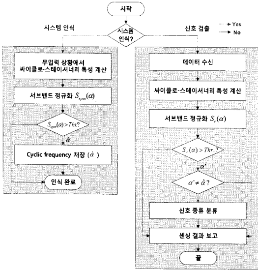
그림 3. 시스템 자체의 스푸리어스가 존재하는 환경에서 오경보 및 미검출 확률을 줄일 수 있는 알고리즘의 순서도
