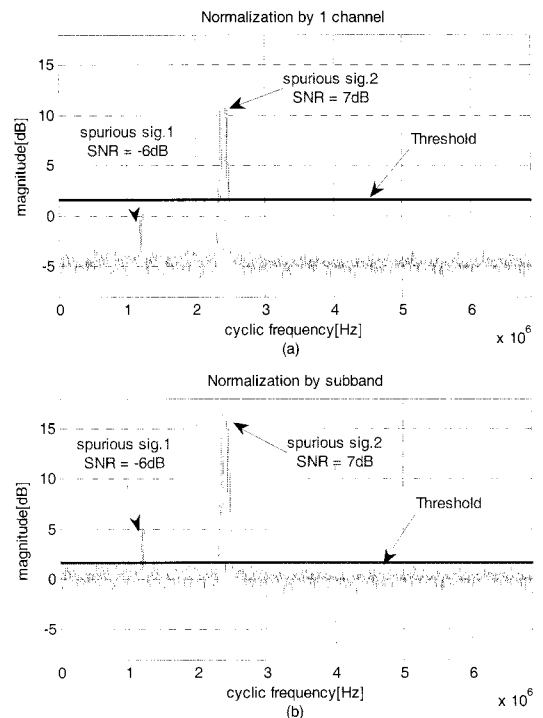
그림 4. 센싱 시스템 내부에 크기가 다른 2개의 스푸리어스 신호가 존재하는 경우 정규화 방법에 따른 사이클로-스테이셔너리 특성 (a) 1 채널 단위로 정규화한 경우의 사이클로-스테이셔너리 특성 (b) 서브 밴드 단위로 정규화한 경우의 사이클로 스테이셔너리 특성
