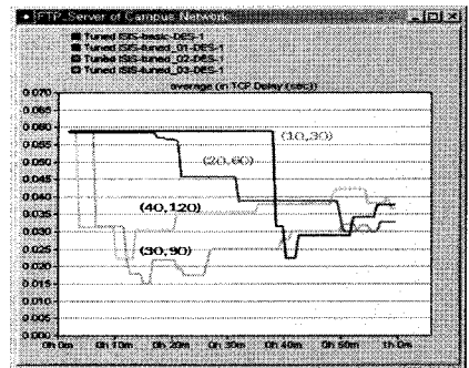
그림 7. FTP: TCP 지연
