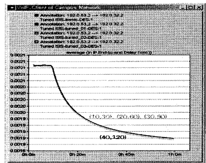
그림 6. VoIP: E-t-E 지연
