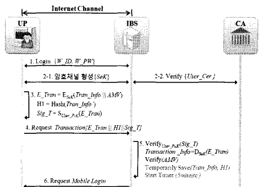
그림 3. 인터넷 채널 통신의 데이터 전송 프로토콜
