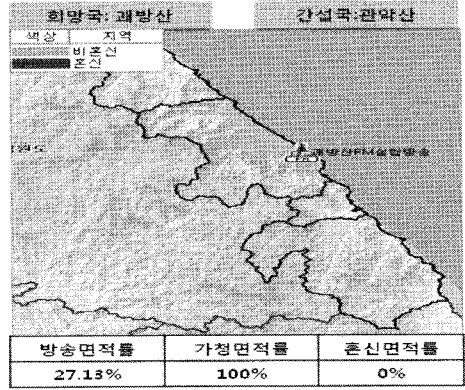
그림 11. 괘방산이 관악산SBS으로부터 받는 간섭 분석 결과 (동일채널 Case 4) Fig. 11. A result of the interference analysis from Mt.Gwan-ak SBS to Mt.Gwae-bang (co-channel Case 4)
