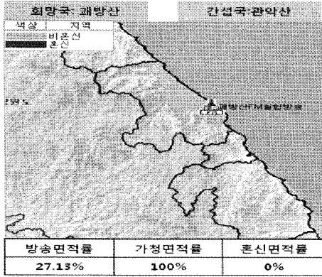
그림 9. 괘방산이 관악산SBS으로부터 받는 간섭 분석 결과 (동일채널 Case 3) Fig. 9. A result of the interference analysis from Mt.Gwan-ak SBS to Mt.Gwae-bang (co-channel Case 3)
