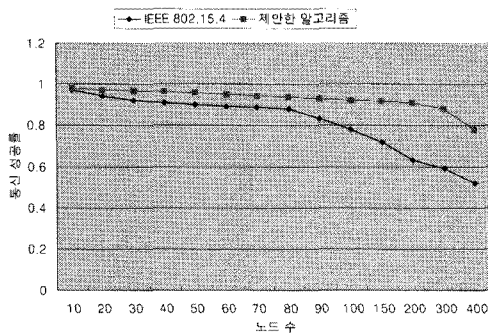
그림 9. PAN 영역 내의 통신 성공률
