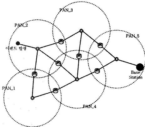
그림 8. 코디네이터와 라우터 노드의 메시 네트워크
