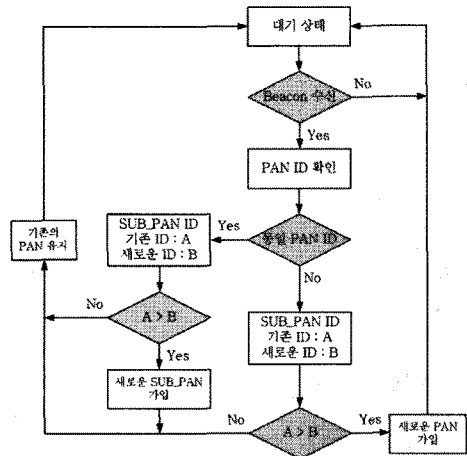
그림 4. 제안하는 노드의 PAN 가입 순서도
