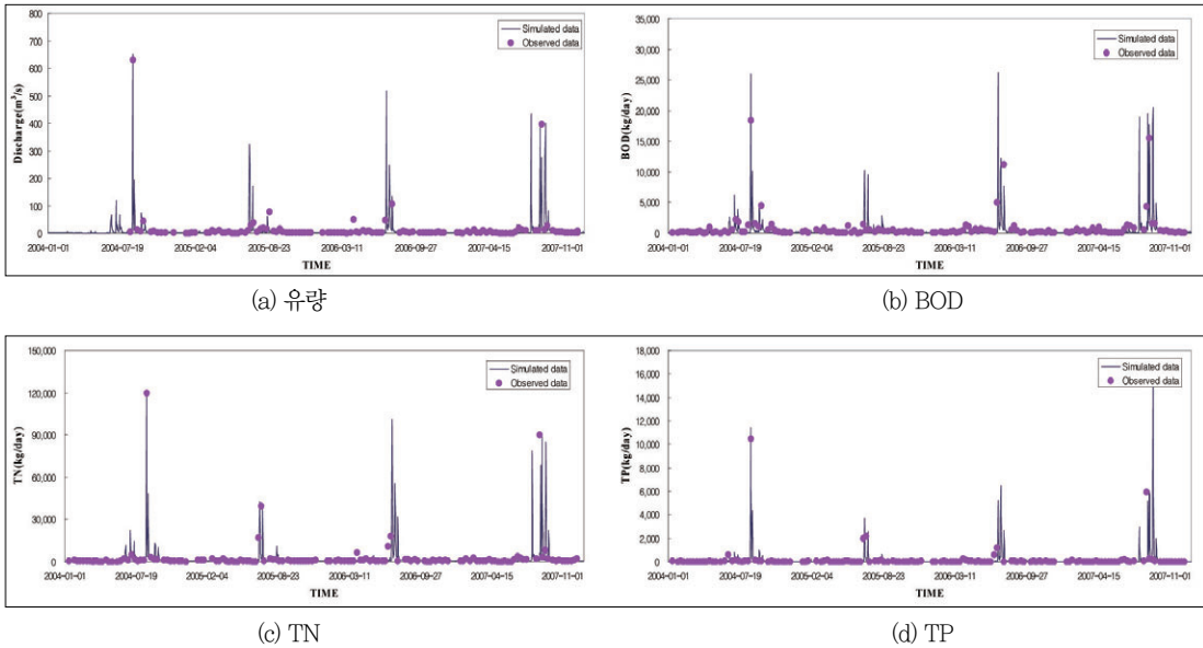
그림 5. 황강 A 유역 모의 결과
