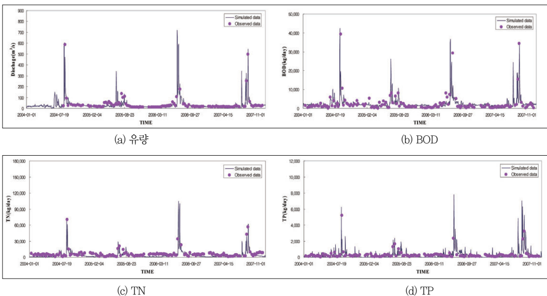
그림 6. 황강 B 유역 모의 결과
