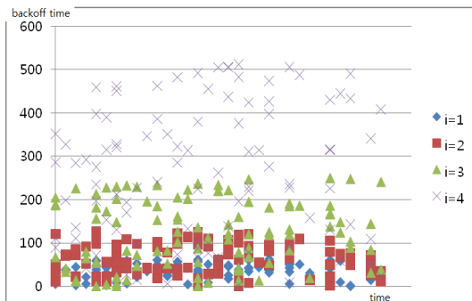
그림 2. 802.11 DCF에서의 백오프시간 분포 Fig. 2 The distribution of the backoff time in the IEEE 802.11 DCF
