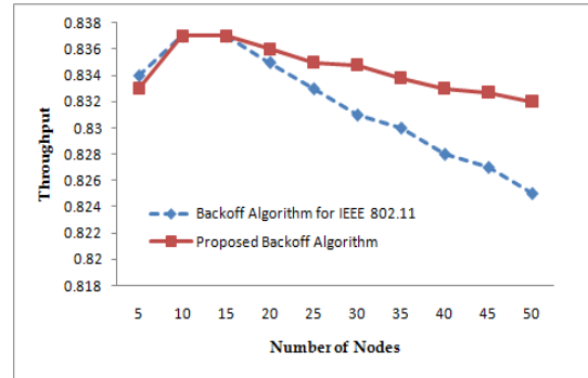
그림 3. 노드 수에 대한 처리율 변화 fig. 3 Throughput vs. number of stations
