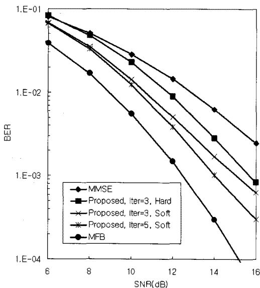
그림 4. 제안된 기법의 BER 성능
