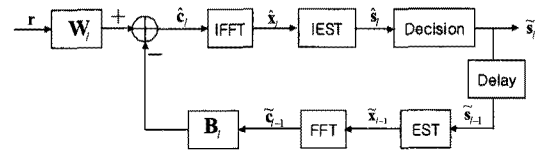
그림 3. 제안된 주파수 영역 반복 등화기
