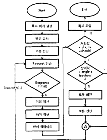
그림 2. Localization 알고리즘
