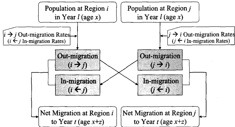
Figure 3. Projection of migration component in a biregional cohort-component method. 이지역 코호트-요인법에서의 인구 이동 추계
