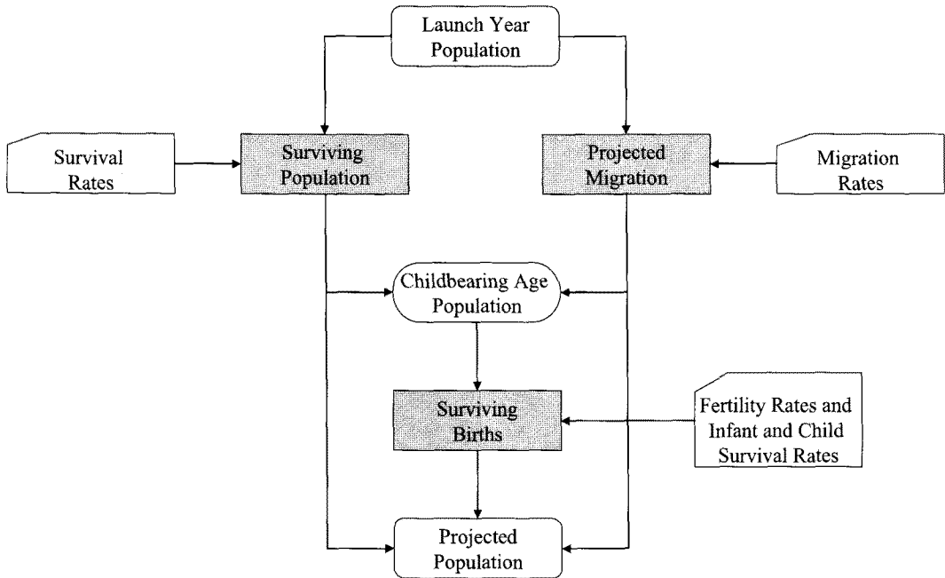
Figure 1. Population projection based on the cohort-component method. 코호트-요인법에 의한 인구 추계 과정 Source: Smith et al. , 2001, 47
