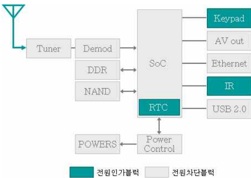
[그림 8] 수동대기 모드시 전원인가 블록
