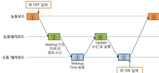
[그림 11] 저전력 셋톱박스 운영 스케줄링 기법
