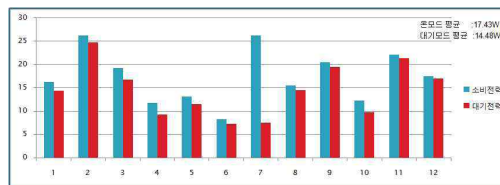
[그림 2] 국내 셋톱박스의 소비전력 비교
