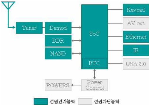
[그림 7] 능동대기 모드시 전원인가 블록
