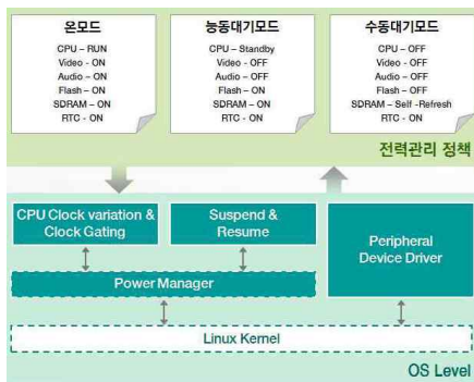
[그림 9] 운영체제 기반의 전력관리정책
