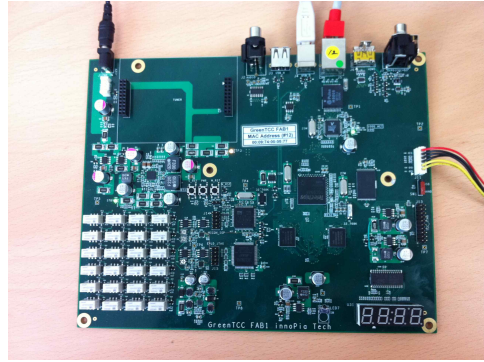
[그림 12] 저전력 셋톱박스 H/W
