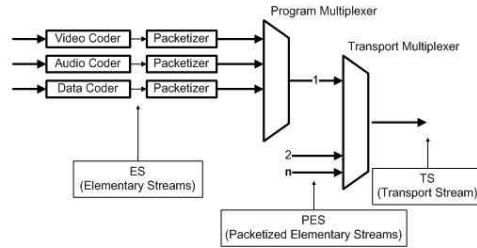
[그림 3] MPEG-2 TS 구조
