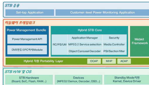
[그림 6] 셋톱박스 전체 구성방안
