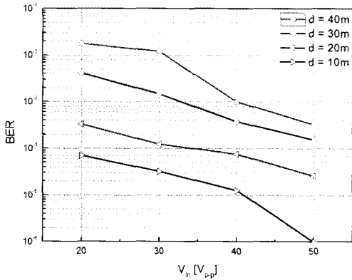
그림 11. 연못에서 송신 모델 트랜스듀서 입력 전압( V_{in} )과 통신 거리( d )에 따른 비트오율 특성
