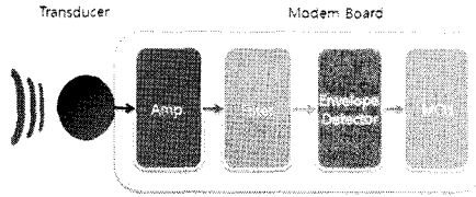
그림 5. 수신부 블록다이어그램
