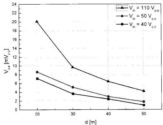
그림 10. 연못에서 송신 모뎀 트랜스듀서 입력 전압( V_{in} )과 통신 거리( d )에 따른 수신 모뎀 트랜스듀서 출력 전압( V_{out} )
