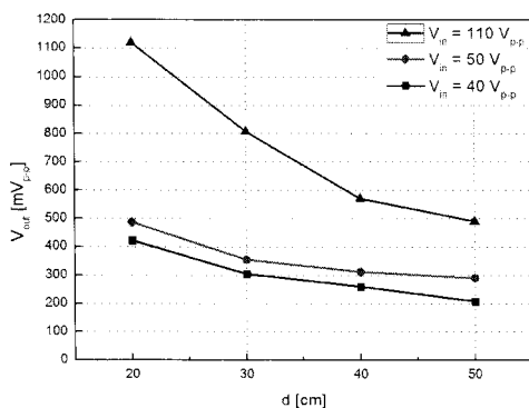
그림 9. 수중에서 송신 모뎀 트랜스듀서 입력 전압( V_{in} )과 통신 거리( d )에 따른 수신 모뎀 트랜스듀서 출력 전압( V_{out} )
