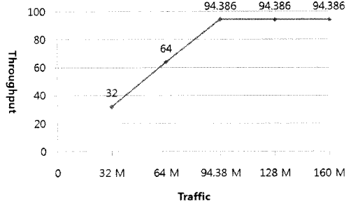
그림 10. 데이터 전송속도 100 Mbps 인 경우의 Data Throughput
