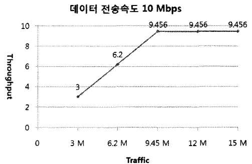
그림 8. 데이터 전송속도 10 Mbps 인 경우의 Data Throughput
