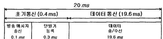
그림 2. 제안하는 프로토콜의 전체 동작시간 할당
