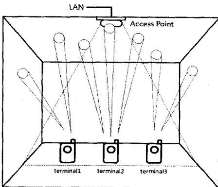
그림 1. LED 조명을 이용한 가시광 통신의 개념도
