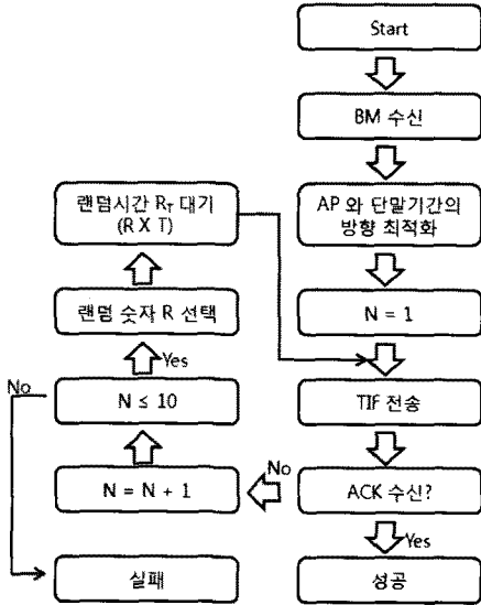
그림 4. 초기통신의 순서도
