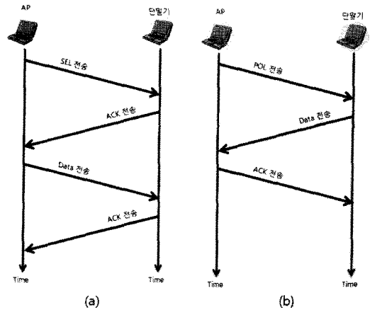
그림 5. 데이터 통신의 흐름도 (a) AP → 단말기 송신할 데이터가 있을 경우 (b) 단말기 → AP 송신할 데이터가 있을 경우
