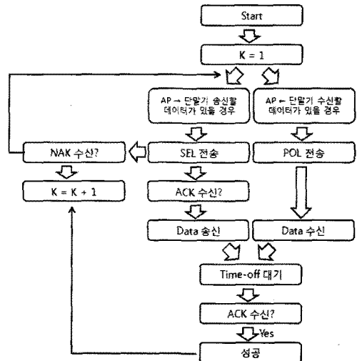
그림 6. 데이터 통신의 순서도
