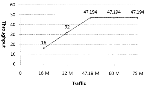
그림 9. 데이터 전송속도 50 Mbps 인 경우의 Data Throughput
