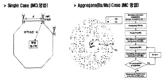
그림 1. C-밴드 위성지구국과 IMT-Advanced 간 간섭 시나리오
