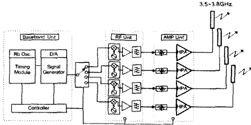
그림 3. 송신 시스템 개요도 Fig. 3. transmission system block
