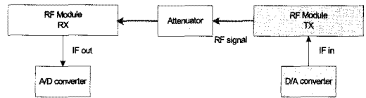
그림 6. back-to-back 측정 시스템의 블록 다이어그램 Fig. 6. back-to-back measurement system block diagram.
