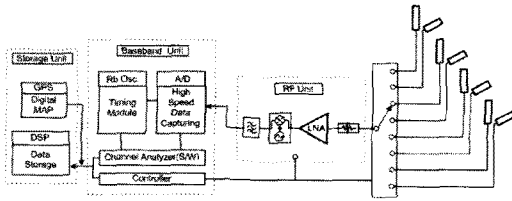
그림 4. 수신 시스템 개요도 Fig. 4. receipt system block
