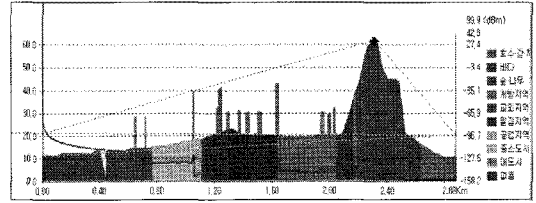
그림 2. 지형/지물에 의한 Path Profile Fig. 2. Ground/shelter for Path Profile
