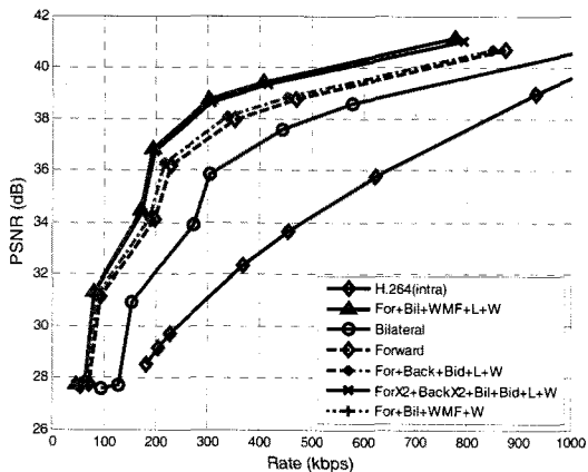
그림 8. 부가정보 생성 기법에 따른 복원된 Wyner-Ziv 영상과 원 영상간의 평균 PSNR 결과 (Foreman)
