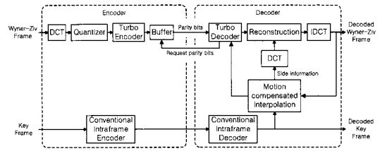
그림 1. 분산 동영상 부호화 시스템의 구조
