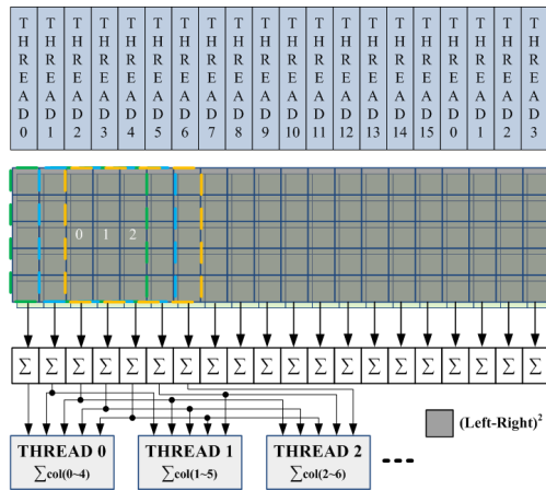
그림 3. 스레드 실행 모델 Fig. 3. Thread execution model
