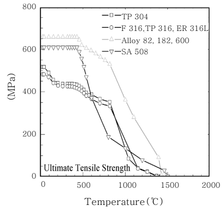
Fig. 12 Tensile strength
