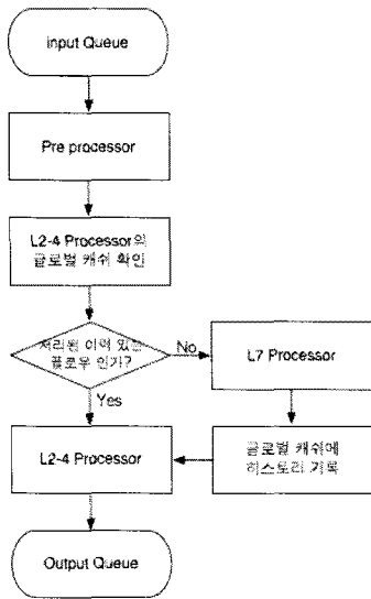
그림 4. 제안된 구조의 패킷 흐름도
