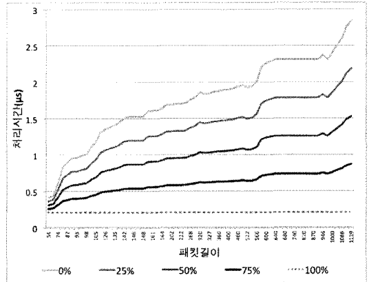
그림 8. 같은 플로우의 패킷이 연속해서 들어올 확률에 따른 L2~4와 L7의 처리 시간
