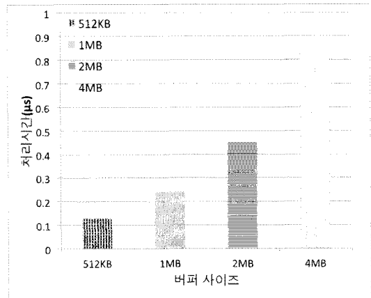
그림 5. L2-4 프로세서의 처리 속도를 EEMBC를 통해서 얻은 결과
