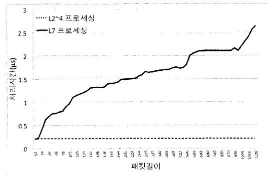
그림 6. L2-4와 L7 패킷 처리시간 비교
