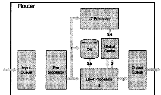
그림 3. 제안된 네트워크 프로세서의 구조
