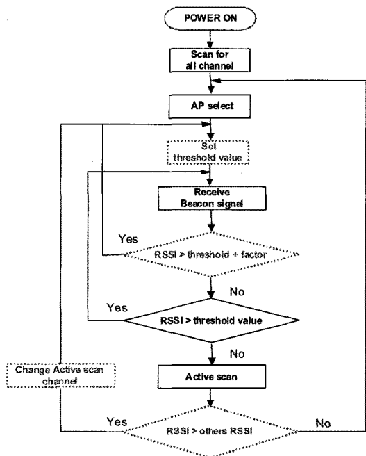
그림 1. 제안하는 핸드오프 알고리즘
