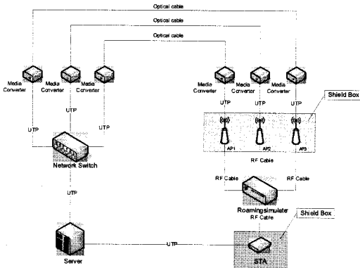
그림 2. 시험을 위한 네트워크 구성
