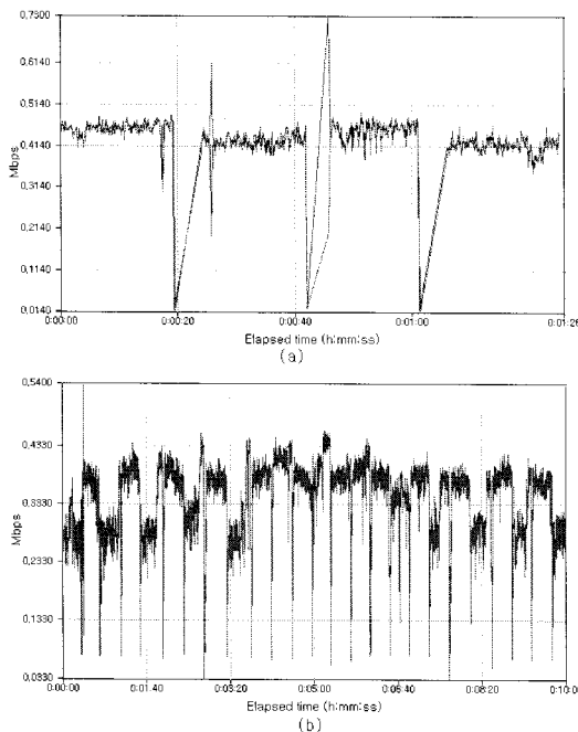
그림 5. 무선 환경이 변할 때 전송률 (a) 일반 무선랜 카드 (b) 알고리즘이 적용된 STA
