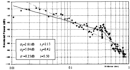
그림 2. LOS 경로에서 측정된 데이터의 단일경사모델과 이중경사모델을 이용한 회귀근사선 (regression fit lines)
