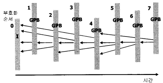
그림 3. 저지연 항목의 GOP 구조
