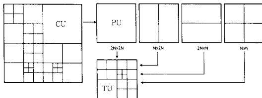
그림 2. HEVC 계층 구조
