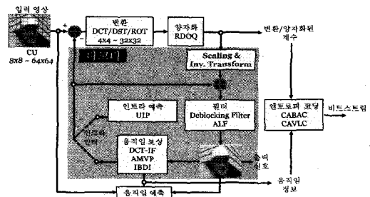
그림 1. HEVC 부호화기 구조
