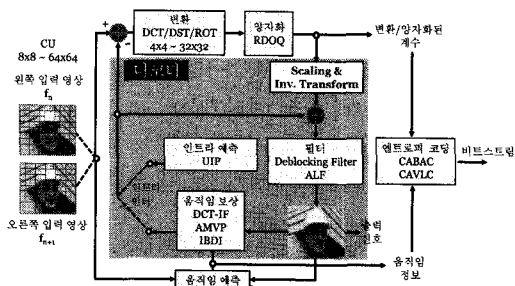
그림 5. HEVC를 이용한 양안식 영상의 부호화기 구조
