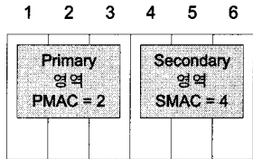
(c) 제안 기술의 bandwidth request 채널 구성
