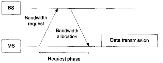
(a) 등급이 높은 사용자의 random access 과정을 통한 자원 요청
