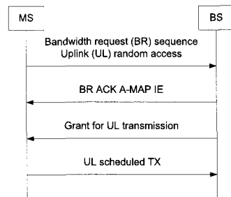
그림 4. Contention-based random access bandwidth request의 동작 과정
