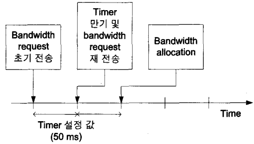
(a) 등급이 높은 사용자의 random access 과정을 통한 자원 요청
