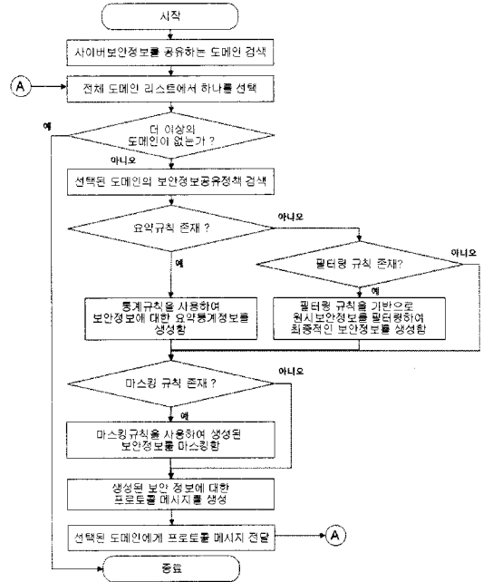
그림 5. 보안정보 공유정책 적용 알고리즘
