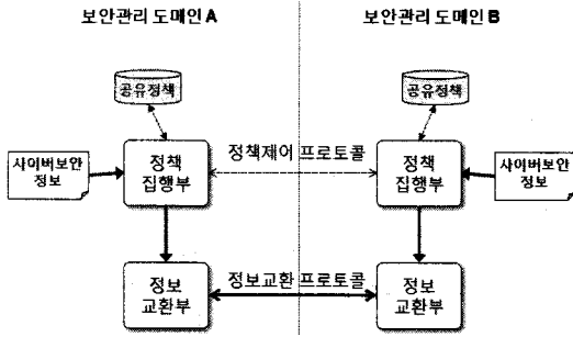
그림 3. 제안하는 사이버보안정보 교환 구조
