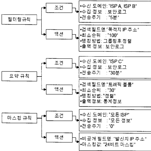
그림 4. 사이버보안 공유정책의 예
