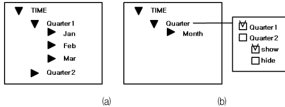
그림 27. 데이터 큐브에서의 탐색 : (a)외연 기반 탐색과 (b)내포 기반 탐색
