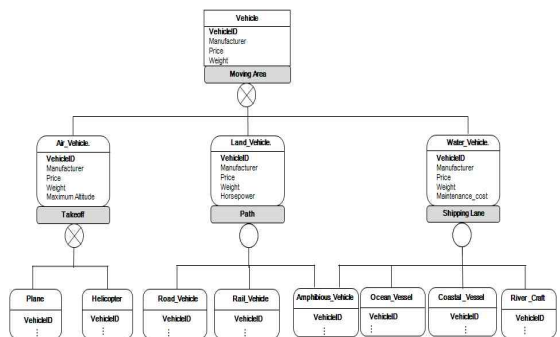
그림 12. 포괄적 계층 Fig. 12. An Inclusive Hierarchy
