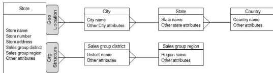
그림 9. 다중기준 계층 Fig. 9. A Multiple Criteria Hierarchy
