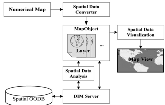
(그림 5) MapObject 시각화
