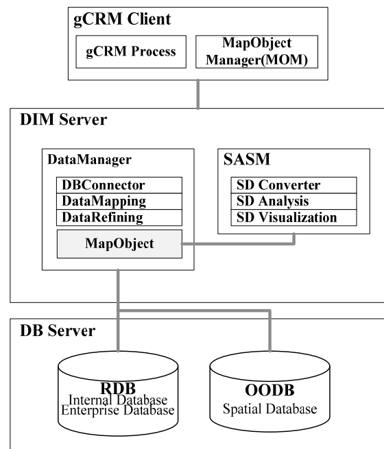
(그림 1) 시스템 구조
