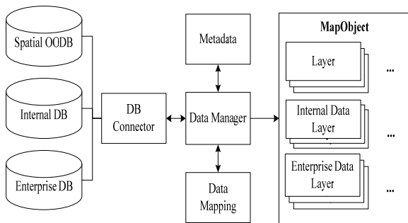
(그림 4) MapObject 생성 과정
