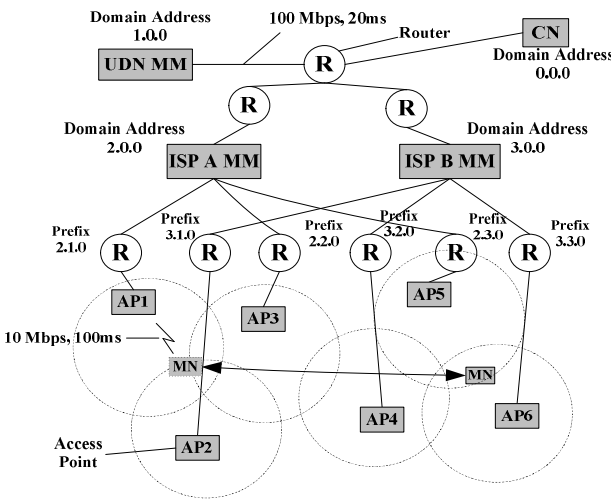
그림 3. 성능 평가를 위한 시뮬레이션 토폴로지 Fig. 3. Simulation topology for performance evaluation.
