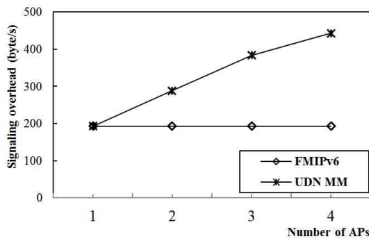
그림 7. IETF FMIPv6와 UDN 프로토콜간 시그널링 오버헤드 비교
