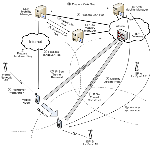
그림 2. UDN을 위한 끊김 없는 이동성 관리를 위한 시나리오
