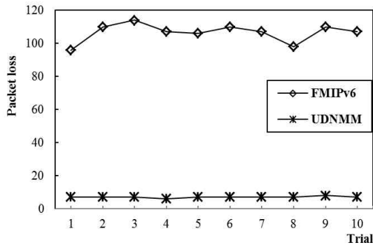
그림 5. IETF FMIPv6과 UDN 패킷 손실 비교 Fig. 5. Comparison of packet loss between IETF FMIPv6 and UDN.
