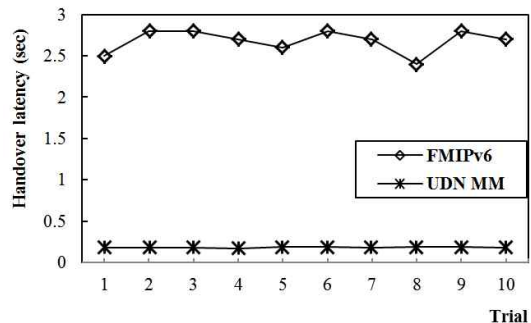
그림 4. IETF FMIPv6와 UDN에 대한 핸드오버 지연시간 비교
