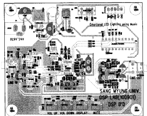
그림 6. 필터방식 DSP 보드
