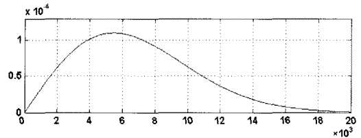
그림 3. 저역 오디오 신호의 pdf
