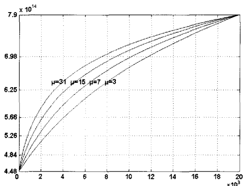
그림 4. \mu 에 따른 저역 주파수 신호의 비선형 매핑 곡선
