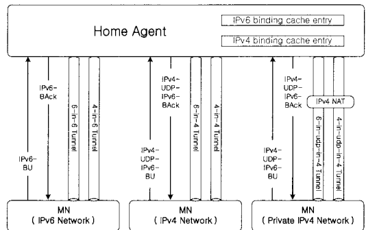
그림 2. DS-MIPv6에서 MN와 HA간의 시그널링 및 터널 설정 방법
