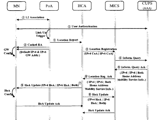
그림 5. AIMS-DS에서 이동단말의 초기 망 접속 절차
