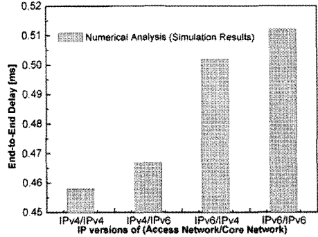
그림 9. AIMS-DS의 패킷 전달 지연시간
