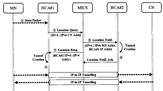
그림 7. AIMS-DS에서 이동단말의 데이터 전송 절차
