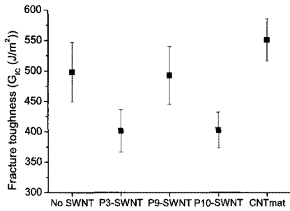
Fig. 5 T700/EPON862/CNT 시편의 모드 1 파괴인성.
