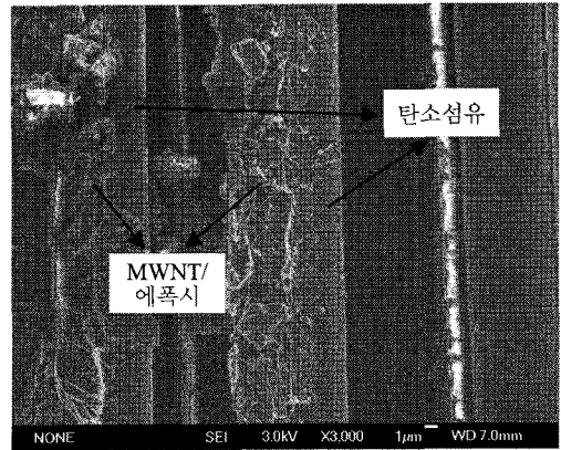
Fig. 7 모드 1 파괴인성 시험 이후 CNT mat 시편의 파단면.
