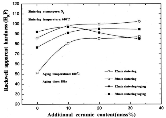
[그림 4] 각 소결체의 겔보기 경도 값(시효처리 전과 후) [Fig. 4] Rockwell apparent hardness(H R F) of various sintered compacts(before and after aging treatment)
