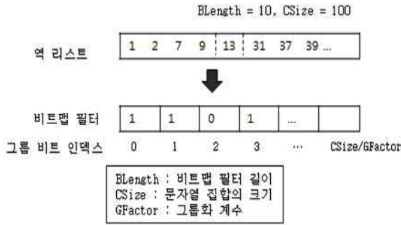
(그림 3) 역 리스트에 대한 비트맵 필터
