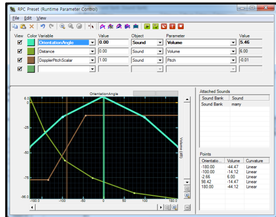
그림 6. RPC 사전설정 Fig. 6 RPC Preset
