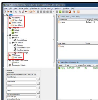
그림 5. XACT v3.0의 기본구조 Fig. 5 Fundamental Structure of XACT v3.0
