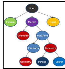
그림 3. Goblin XNA의 노드구조 Fig. 3 Goblin XNA Scene Graph Hierarchy
