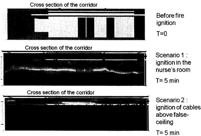
[그림 4] 화재모델링 결과
