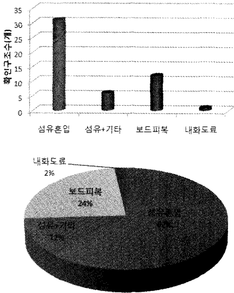
그림 4. 성능확인구조의 내화대책 분포
