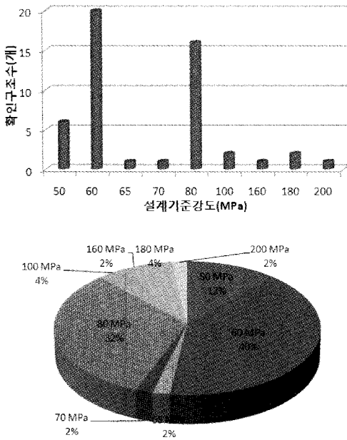
그림 3. 성능확인구조의 설계기준강도 분포
