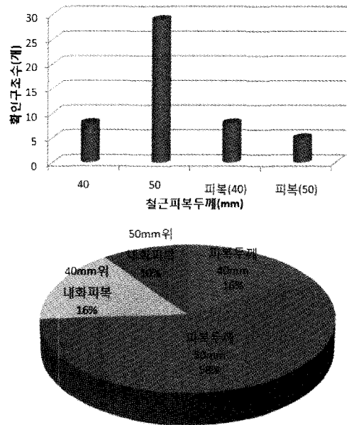
그림 5. 성능확인구조의 콘크리트 피복두께 분포
