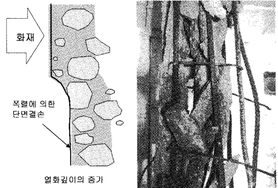
그림 1. 폭렬현상 발생 및 시험예
