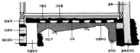
〈전통 방식의 온돌 구조도〉
