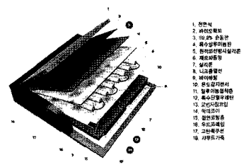
〈온돌식 전기침대 내부구조 예〉
