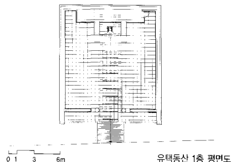
유택동산 1층 평면도
