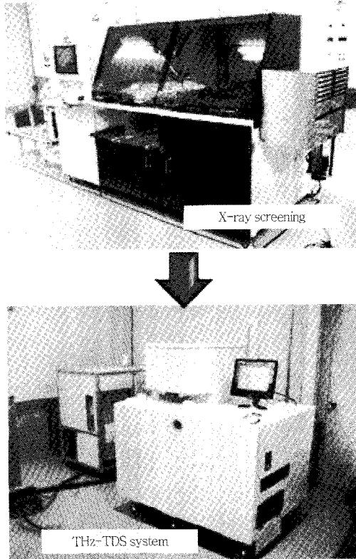
(그림 6) 일본 RIKEN의 2단계 우편물 검색장치. 1차 X-선 검사와 2차 테라헤르츠 검사를 거쳐 위험물을 검색
