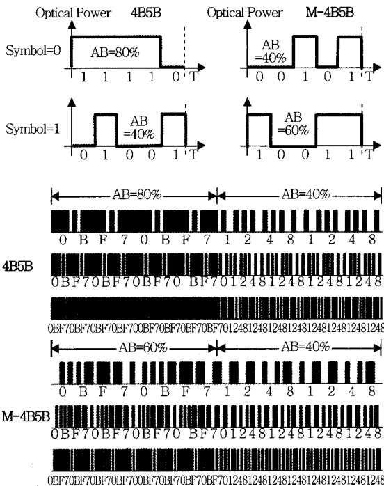
(그림 8) 가시광 무선통신에서 4B5B 코드와 M-4B5B 코드 적용에 따른 광 출력 파형의 비교 예 (AB=Average Brightness)[6],[13]
