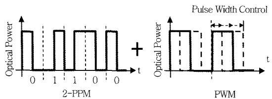
(그림 13) Variable-PPM 변조 방법의 원리[6]-[8]
