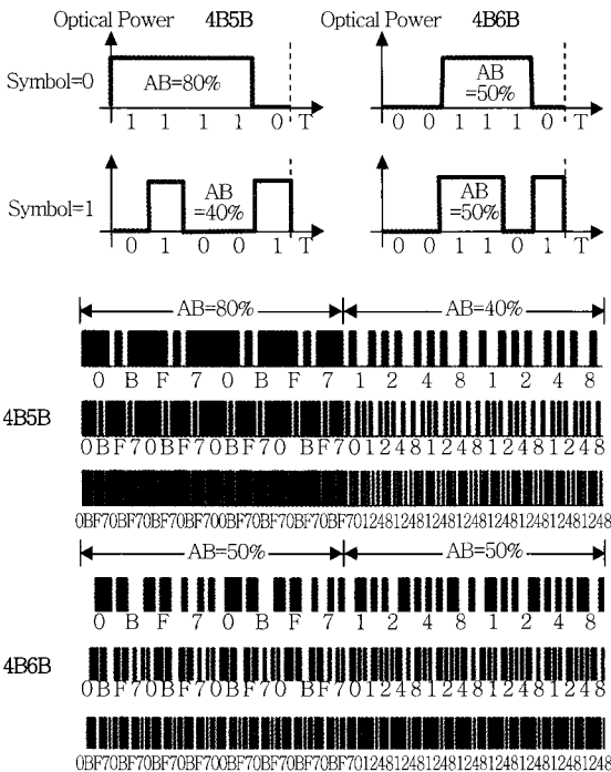
(그림 10) 가시광 무선통신에서 4B5B 코드와 4B6B 코드 적용에 따른 광 출력 파형의 비교 예 (AB=Average Brightness)[6],[13]
