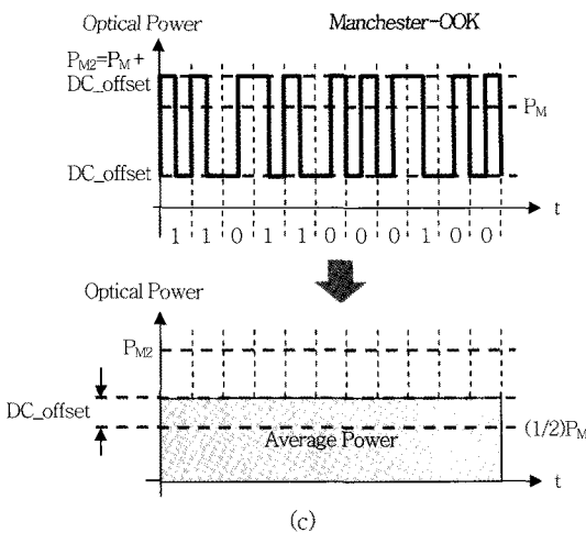
(그림 12) Manchester-OOK 환경에서의 'Amplitude Dimming'[6],[7]
