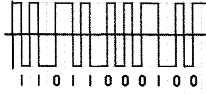
(그림 5) Manchester 코드의 부호화 예[12]
