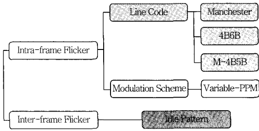
(그림 4) 플리커 방지를 위한 가시광 무선통신 기술 [6],[10]
