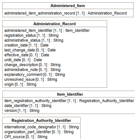
그림 6. 관리 영역 메타모델 Fig. 6. The Administration region metamodel
