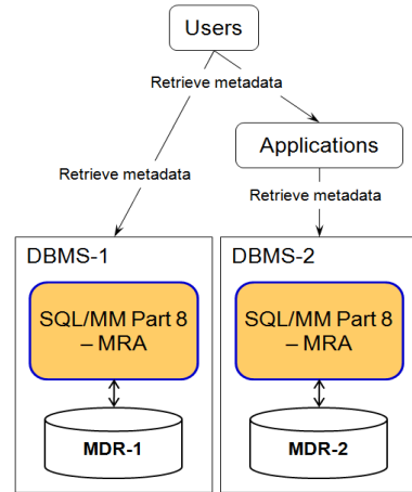
그림 4. 전체적인 프레임워크 Fig. 4. Overall framework
