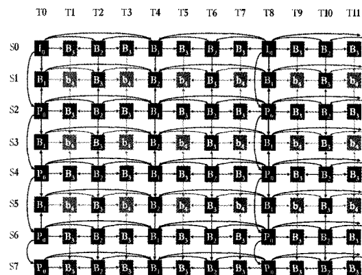
그림 7. 계층적 B화면을 이용한 기본적인 예측 구조
