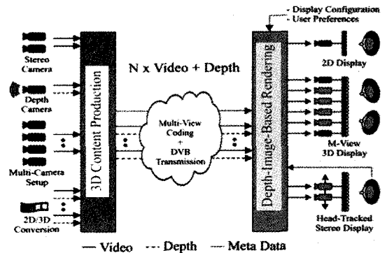
그림 4. 다시점 영상을 이용한 3차원 비디오 시스템
