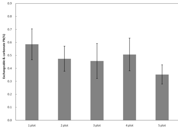
(a) Exchangeable 및 carbonate 아연의 분획특성
