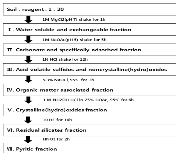
그림 7. 토양 내 비소의 연속분획 분석절차(La Force 등, 2000)
