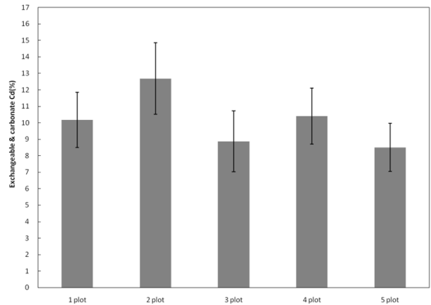
(b) Exchangeable 및 carbonate 카드뮴의 분획특성
