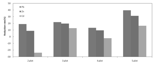
그림 13. 교환성(exchangeable) 및 탄산염결합 형태(carbonate) 중 금속 성분의 저감율
