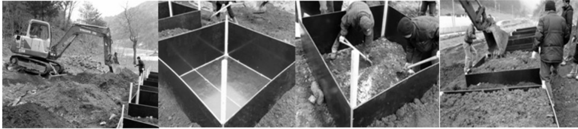
그림 4. 현장실증시험 처리구 설치 전경
