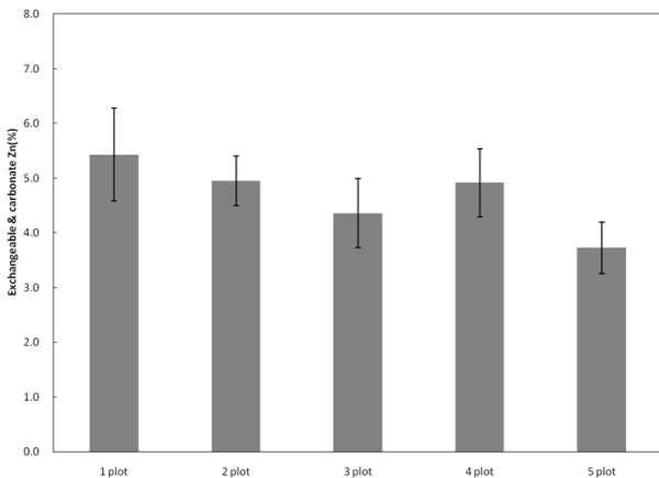
(c) 각 처리구별 Exchangeable 및 carbonate 납의 분획특성
